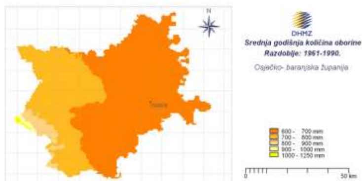
Slika 5.22 – Srednja godišnja količina oborina (mm) u Osječko-baranjskoj županiji od 1961. do 1990. godine
