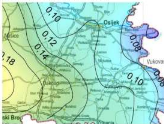
Slika 5.3 – Seizmološka karta horizontalnih akceleracija u povratnom razdoblju 475 godina
