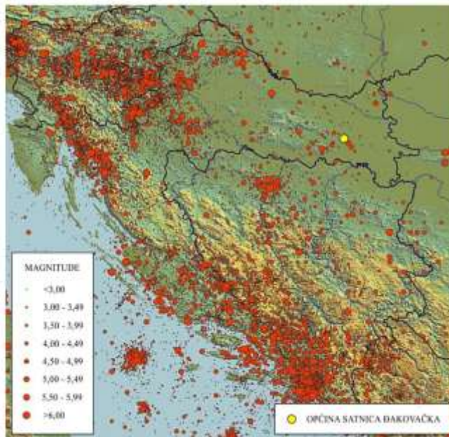
Slika 5.2 – Prikaz epicentara i intenziteta potresa u zadnjih 100 godina
